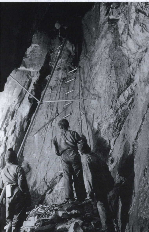
Maszt składany w Jaskini Zimnej, 09. 1953 r.
